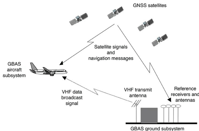
Figura 3.11: Principio operativo de GBAS [Fig14].
